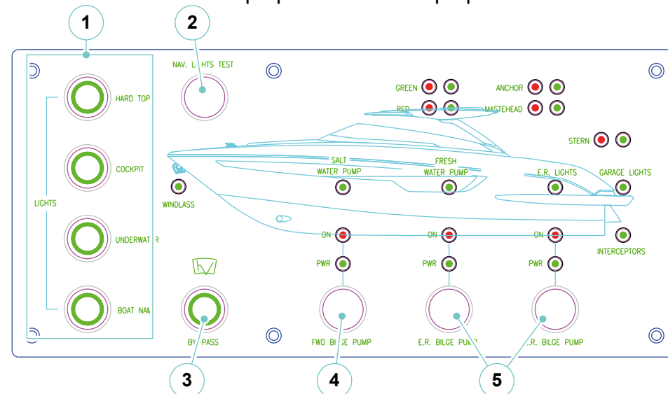
Versione hard top optional / Hard top optional version
