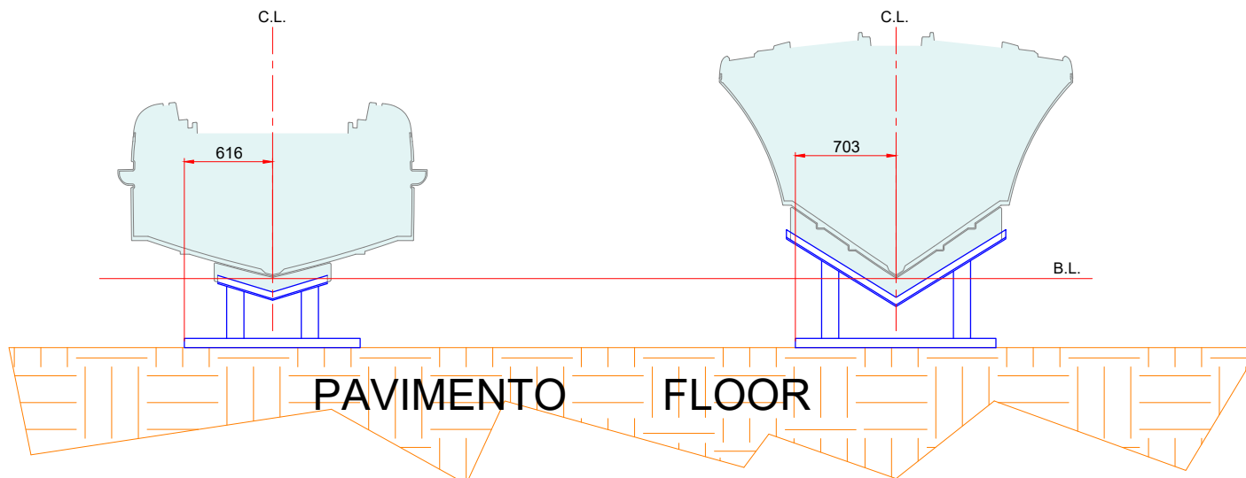
SEZIONE TRASVERSALE (POPPA) CROSS-SECTION (STERN)
