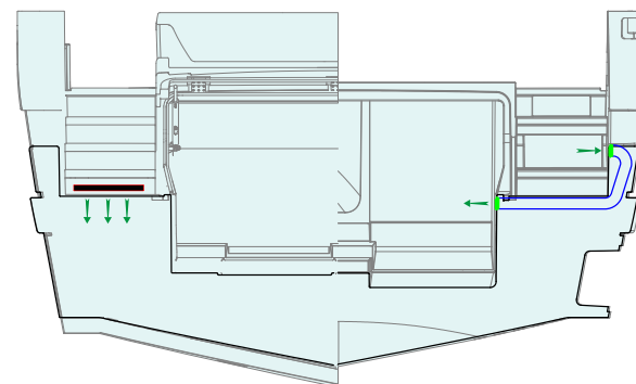
VENTILAZIONE VANO GARAGE GARAGE VENTILATION
